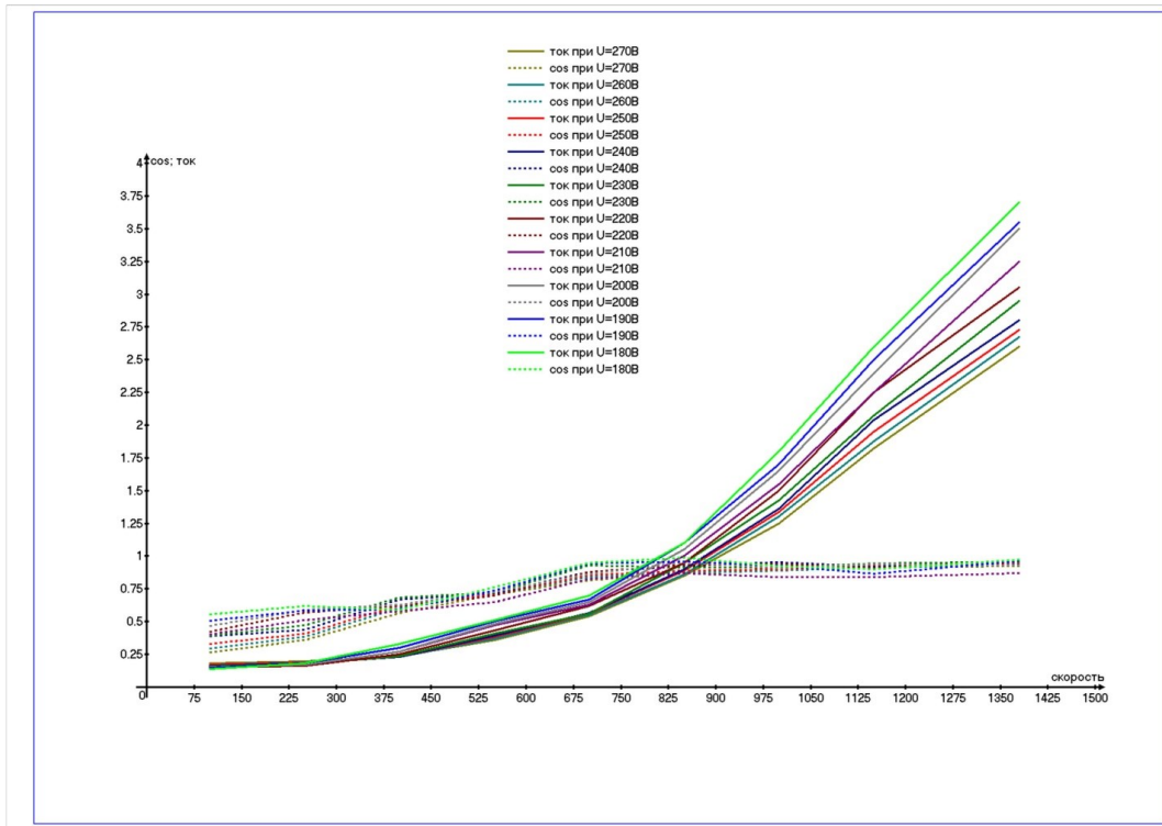
Рис. 5 Зависимость тока и коэффициента активной мощности от скорости вращения при изменении напряжения
