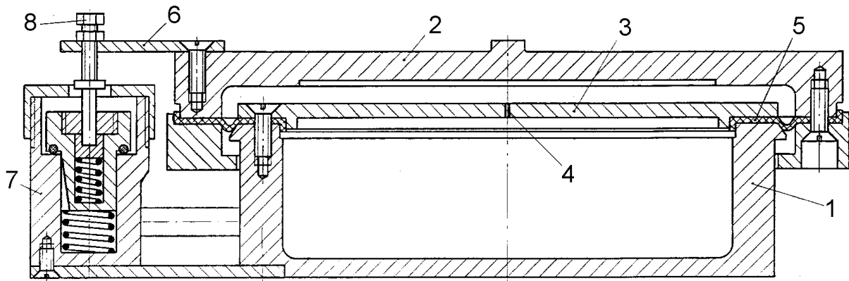
Рис. 3 Конструктивная схема пневматической виброизолирующей системы: 1— корпус; 2—крышка; 3—перегородка; 4—межкамерный дроссель; 5—эластичная диафрагма; рычаг обратной связи; 7— автоматический регулятор уровня; 8— регулировочный винт
