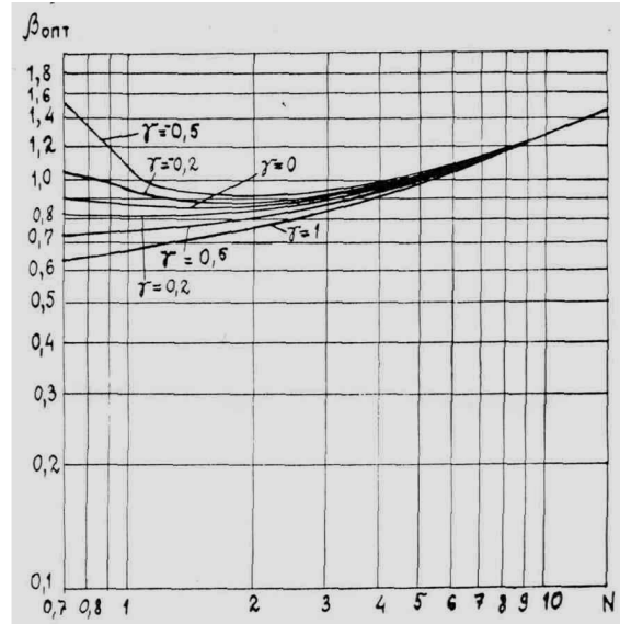
Рис. 3 Графики b_{\text{опт}} = f(N) , изображенные на рис.5, рассчитаны для значений g = 0,2 ; g = 0,5 ; g = 1 ; g = -0,2 ; g = -0,5 дают возможность определить значения оптимального демпфирования для различных g .
