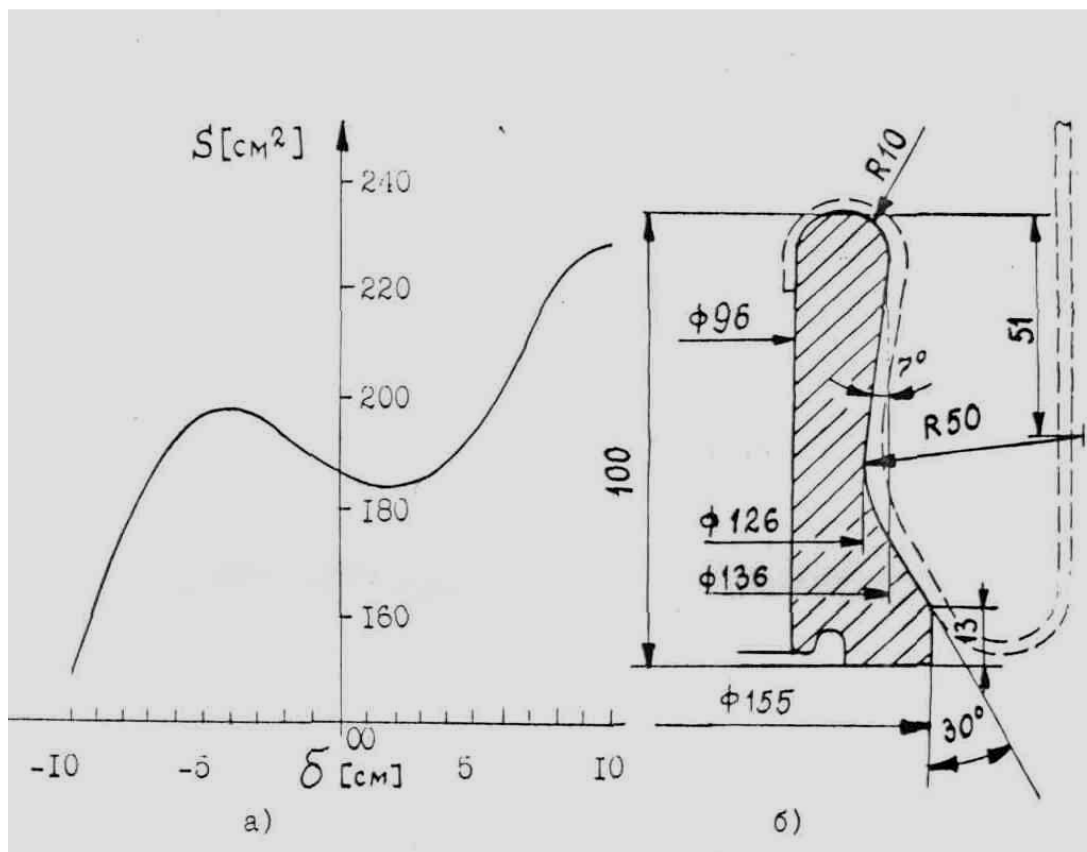
Рис. 4 Характеристики рукавных РКО: а) график жесткость s_1 , стремящийся к нулю и отрицательному значению, б) конструктивная схема введения в РКО обтекателей, которые формируют упругую характеристику при накатывании рукава
