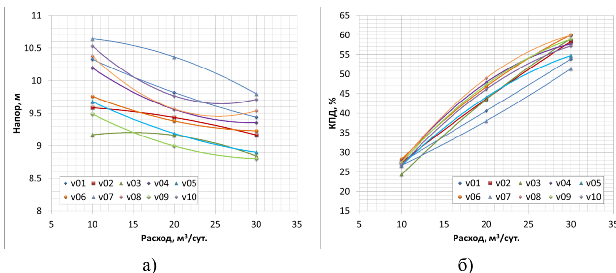
Рис. 4 Рабочие характеристики насосного агрегата а) напор, б) КПД
