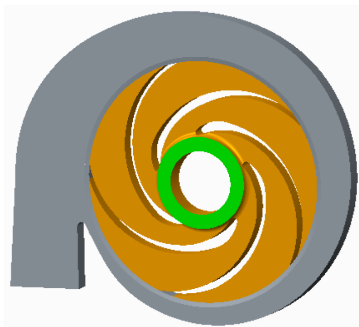
Рис. 1 Модель проточной части модифицированного насосного агрегата
