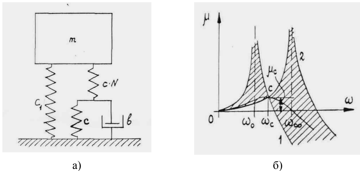
Рис. 1 Система виброизоляции с пневматической пружиной на основе РКО: а) схема механического аналога, б) график коэффициента передачи.
