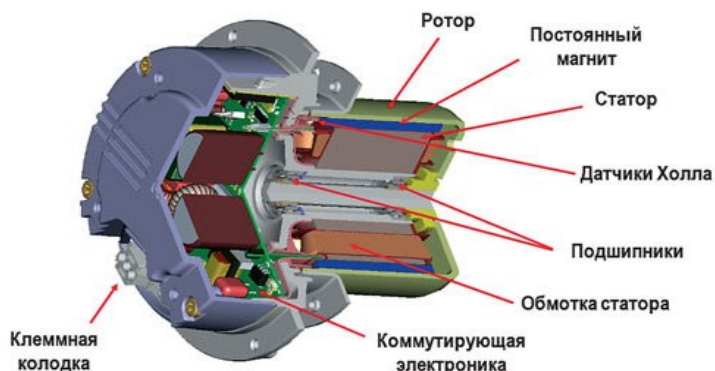
Рис. 1 Устройство энергосберегающего ЕС-двигателя
