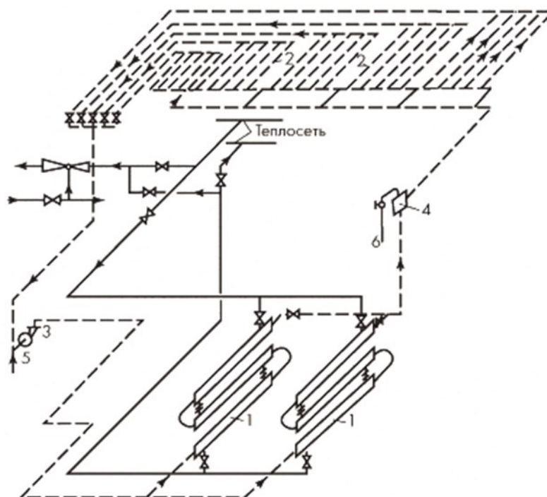
Рис. 1 Схема установки с теплоносителем антифризом
