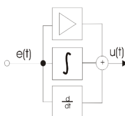
Рис. 3 Схема, иллюстрирующая принцип работы ПИД-регулятора
