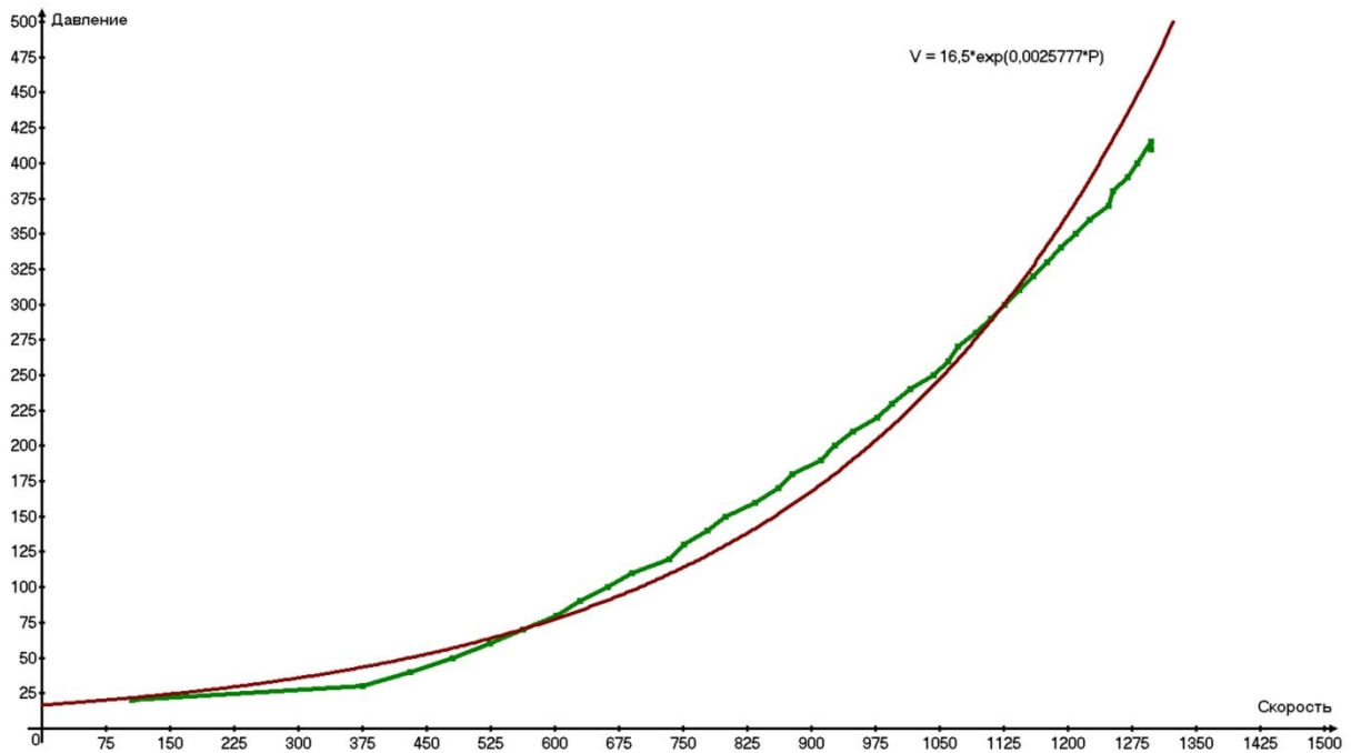
Рис. 6 Зависимость скорости вращения от создаваемого вентилятором давления
