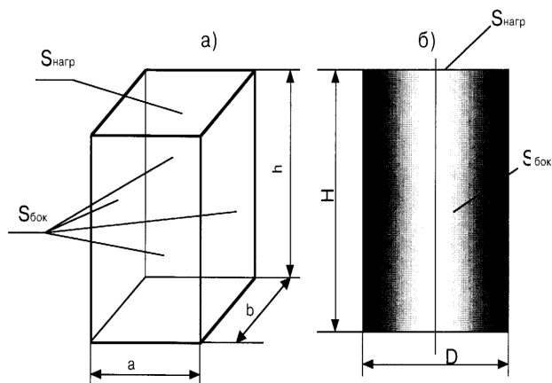
Рис. 4 Расчетные схемы упругих резиновых элементов виброизоляторов: а) призматического; б) цилиндрического.
