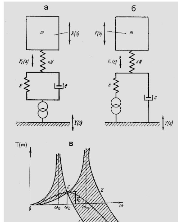
Рис. 2 Эквивалентные линейные модели пневмовиброизоляторов по схемам I и II, (а и б) и коэффициенты передачи пневматической вибро-защитной системы с оптимальным демпфированием (в)
