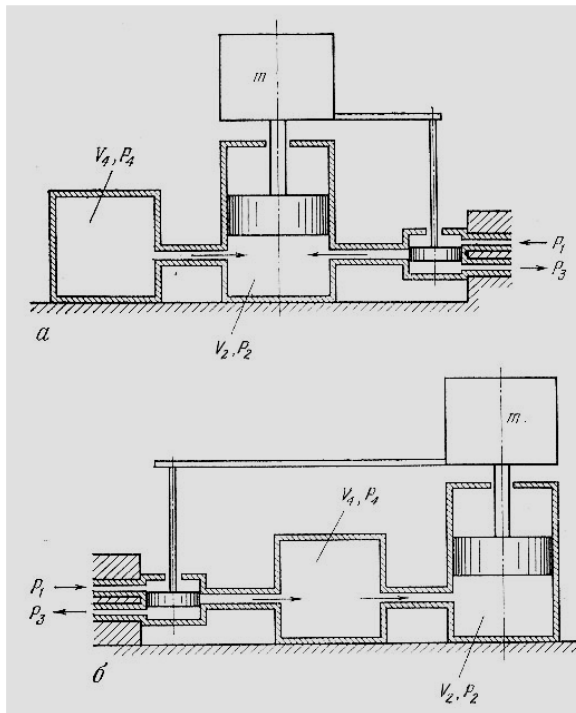
Рис. 1 Типовые схемы пневматических виброизоляторов: а – схема I с регулятором, присоединенным к демпферной камере; б – схема II с регулятором, присоединенным к рабочей камере
