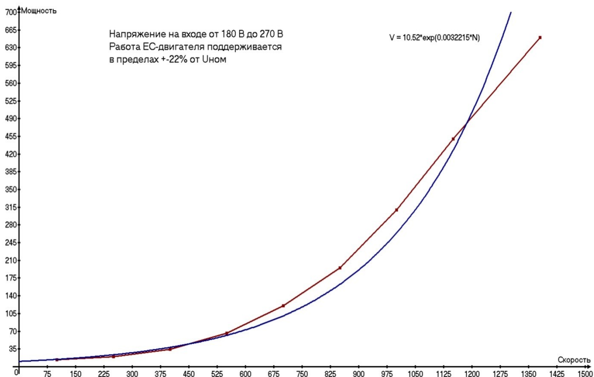
Рис. 7 Зависимость скорости вращения от потребляемой мощности
