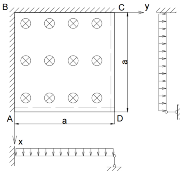
Рис. 1 Расчетная схема
