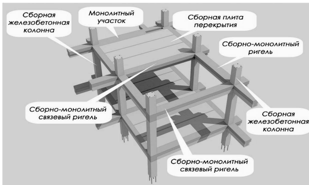
Рис. 1 Схема сборно-монолитного каркаса здания
