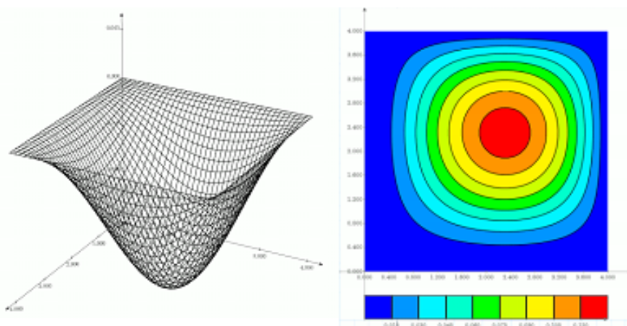
Рис. 2 Объемное изображение полученных прогибов. График прогибов
