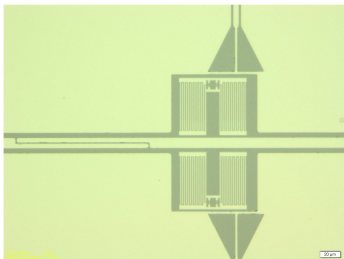
Рис. 1 Два трансмона вблизи сверхпроводящего резонатора. Созданные с помощью технологии двухуглового теневого напыления. Изображение получено с помощью оптического микроскопа
