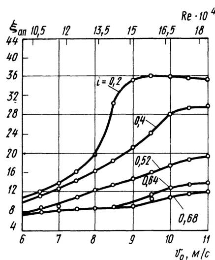
Рис. 6 Зависимость коэффициента сопротивления аппарата \xi_{ап} от скорости движения воздуха в контактно-выхлопной трубе v_0 и относительного уровня жидкости в нем при различном соотношении i = b_p / d_{тр} ( d_{тр} = 250 мм)
