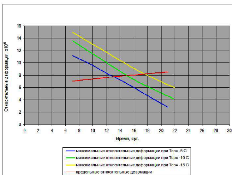
Рис. 1 Результаты исследования деформаций на поверхности блока бетонирования при температурах -5 , -10 и -15\text{ }^{\circ}\text{C}
