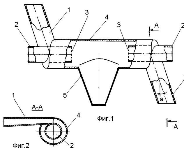
Рис. 1 I-я ступень очистки: вихревой пылеуловитель
