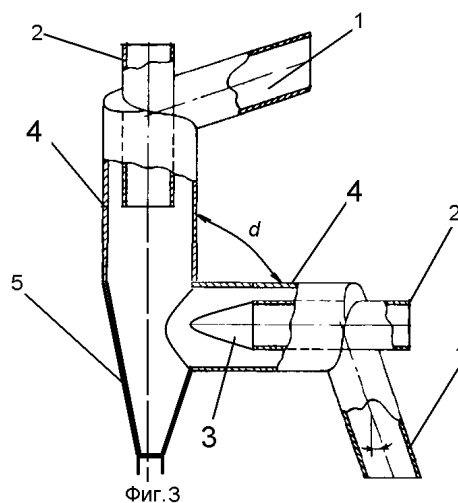
Рис. 2 I-я ступень очистки: вихревой пылеуловитель
