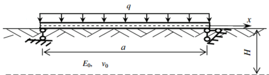
Рис. 1 Общая расчетная схема плиты на упругом основании с действующими нагрузками
