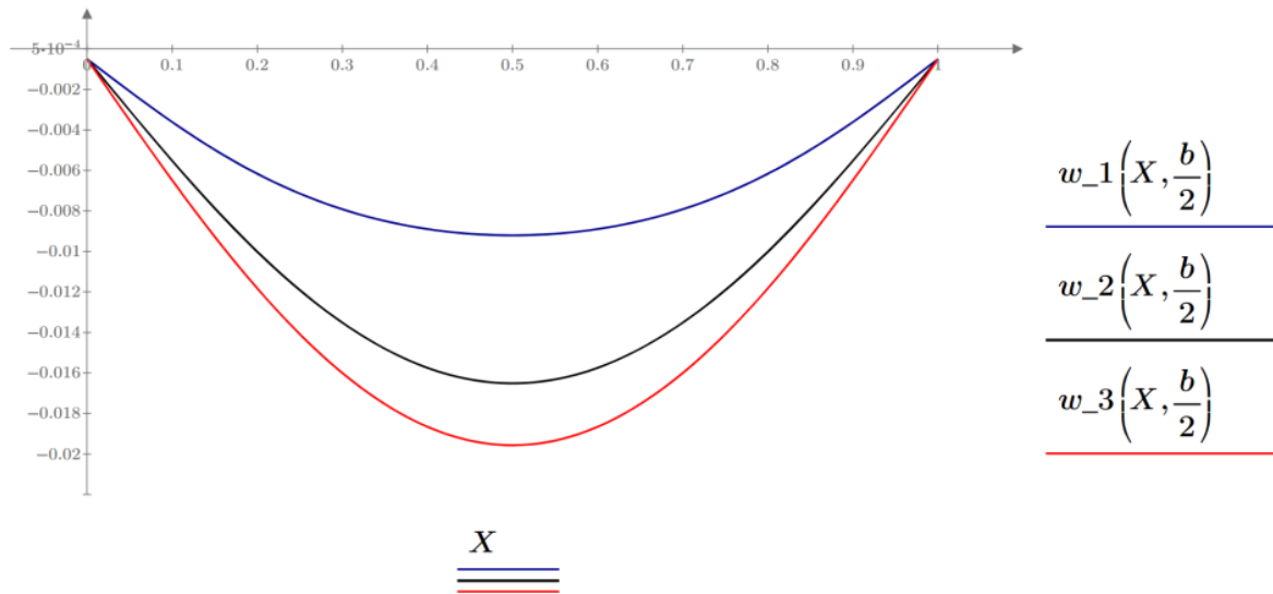
Рис. 2 Схема перемещений при разных способах расчета w_1(x,y) – перемещение при учете упругого основания; w_2(x,y) – перемещение с учетом геометрической нелинейности; w_3(x,y) – перемещение линейной задачи
