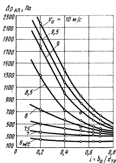
Рис. 5 Зависимость перепада давления от относительного уровня жидкости в нем, определяемом соотношением i = b_p / d_{тр} и скорости движения воздуха в контактно-выхлопной трубе v_0 ( d_{тр} = 250 мм)
