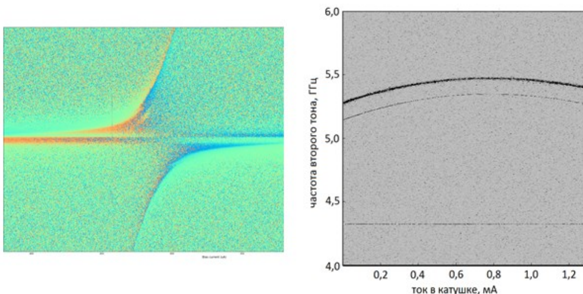
Рис. 2 Слева: Антикроссинг. Результат расщепления уровней кубита и резонатора. Справа: спектр кубита, полученный с помощью двухтоновой спектроскопии. Горизонтальная линия внизу – резонатора, две дуги сверху – резонансные частоты кубита, зависящие от приложенного магнитного поля
