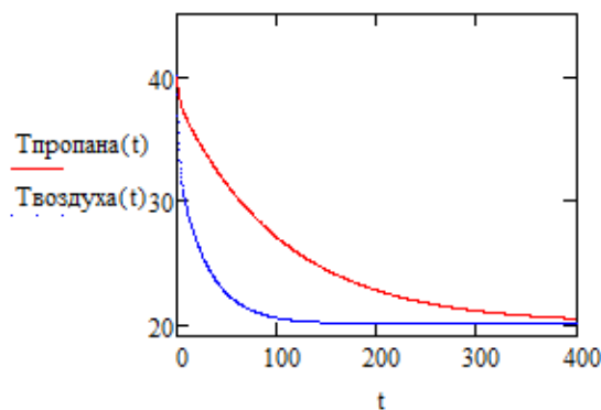
Рис. 2 Процесс охлаждения газов
