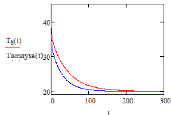
Рис. 4 Процесс остывания смеси газов в сравнении с чистым воздухом
