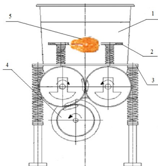
Рис. 1 Лабораторная установка для посола рыбы в поле механических колебаний
