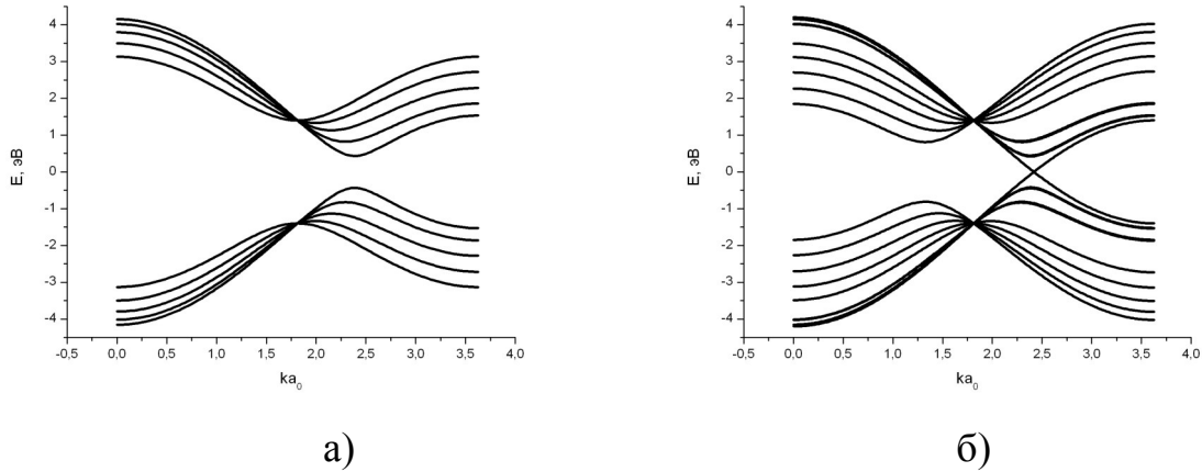
Рис. 2 Дисперсионные кривые двухслойной графеновой наноленты шириной N=5 гексагонов с учетом приложенной тангенциальной компоненты внешнего электрического поля: а) E_\tau = 0 В/мкм, б) E_\tau = 29,2 В/мкм, в) E_\tau = 87,4 В/мкм.
