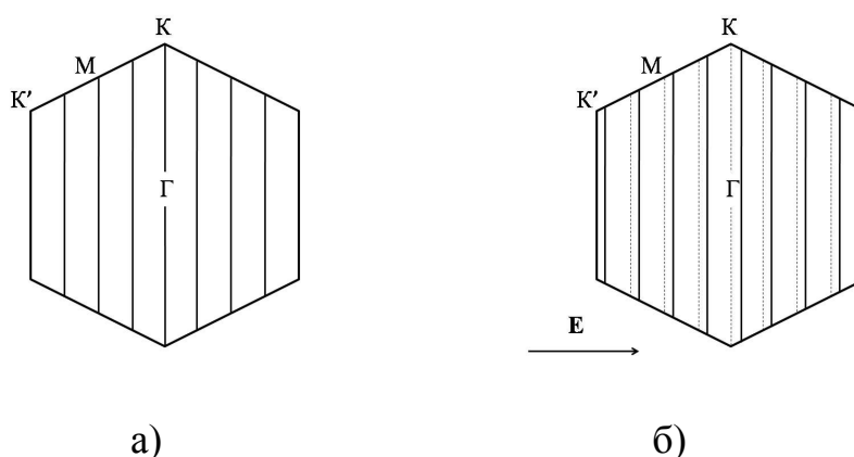
Рис. 3 Разрешённые значения k векторов в зоне Бриллюэна для графеновой наноленты: а) в отсутствии внешнего электрического поля, б) во внешнем электрическом поле E .
