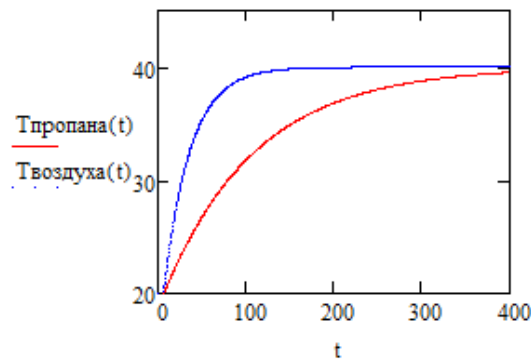
Рис. 1 Процесс нагревания газов
