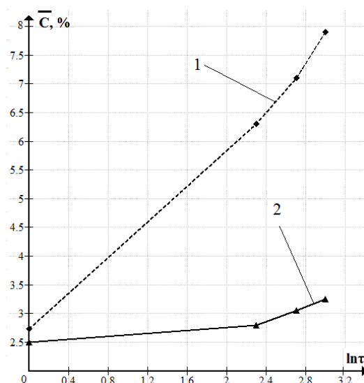
Рис. 4 Сравнение графиков измерения средней солености горбуши при посоле. 1 – под вибрацией и различающимся режимом колебаний рассола и продукта; 2 – при традиционном
