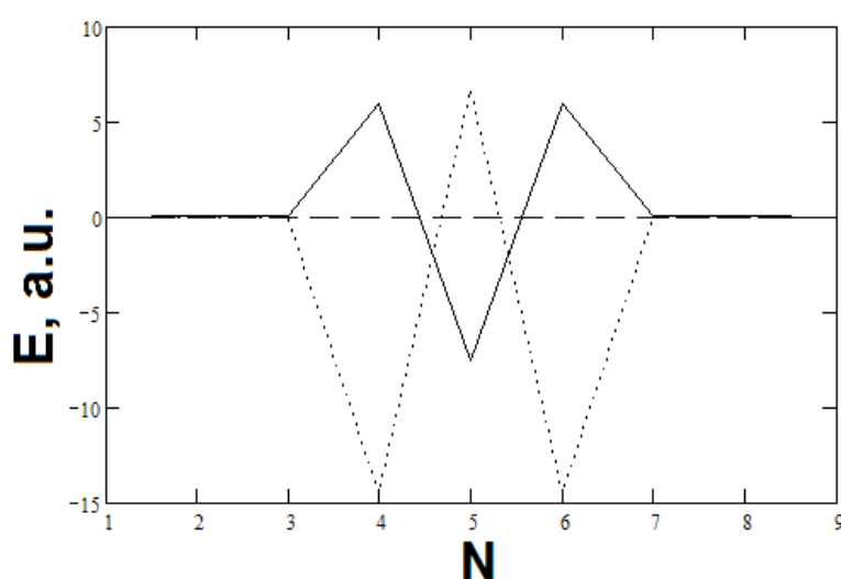
Рис. 1 Зависимость электрического поля, определяемого потенциалом в уравнении (9) от номера волновода. По оси x номер волноводов N , по оси y безразмерная величина электрического поля (единица соответствует 10^8 В/м). Для сплошной кривой - t=130 (единица соответствует 3 \cdot 10^{-16} с), для точечной кривой t=200 , для пунктирной t=260 , W=3.0 , \beta=1
