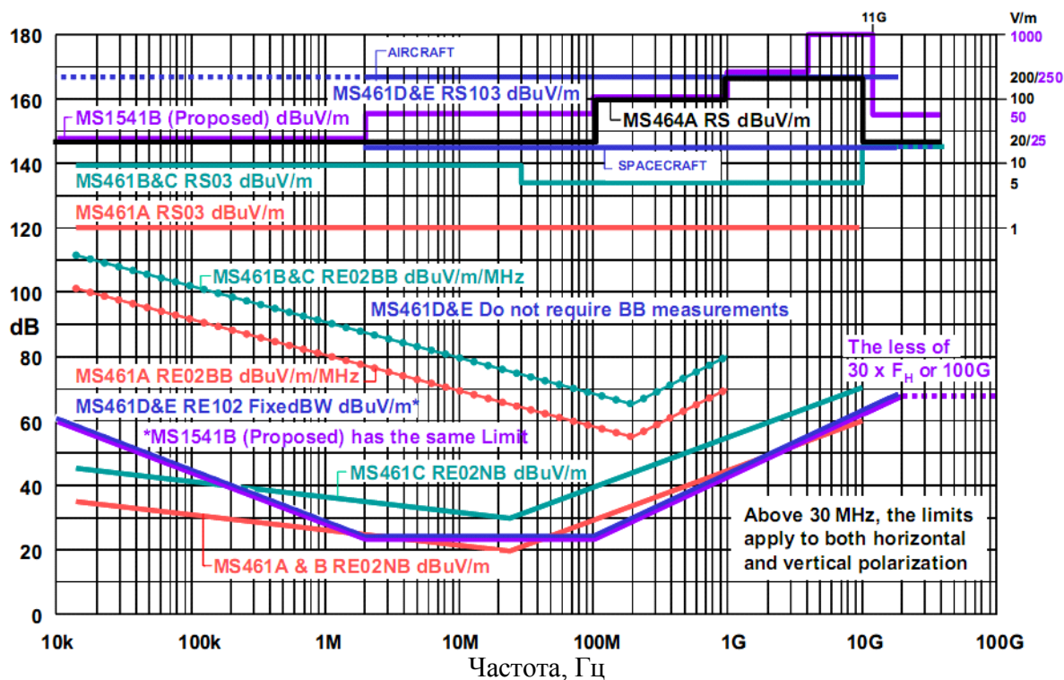
Рис. 1 Сравнение пределов MIL-STD-461A, B, C, D, E; 464A; 1541B, излучаемые эмиссии и восприимчивость к излучаемым эмиссиям
