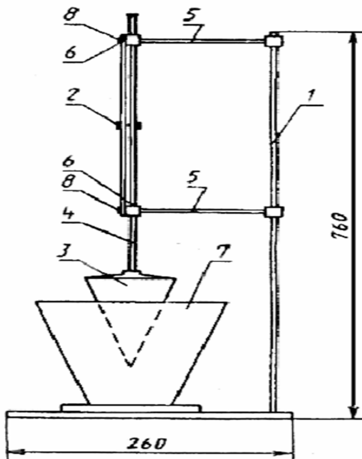
Рис. 1 Прибор для определения подвижности растворной смеси: 1 - штатив; 2 - шкала; 3 - эталонный конус; 4 - штанга; 5 - держатели; 6 - направляющие; 7 - сосуд для растворной смеси; 8 - стопорный винт
