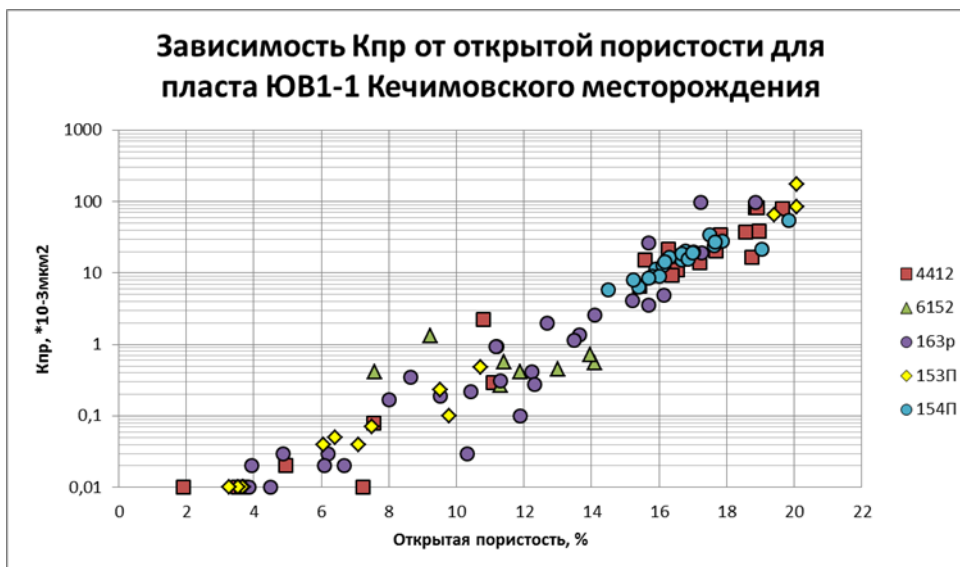
Рис. 1 Зависимость Кпр от открытой пористости для пласта ЮВ 1 1 Кечимовского месторождения
