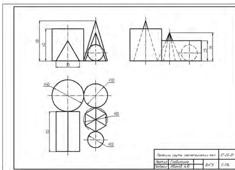
Рис. 4 Проекции группы геометрических тел
