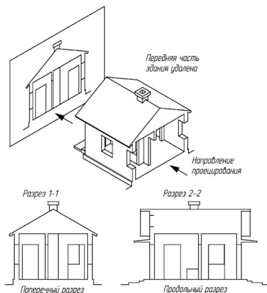
Рис. 3 Проекции дома
