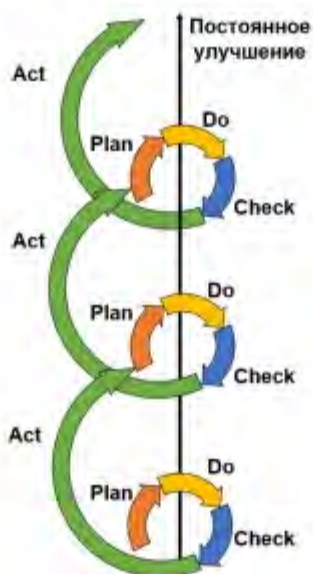
Рис. 2 Спираль Джурана
