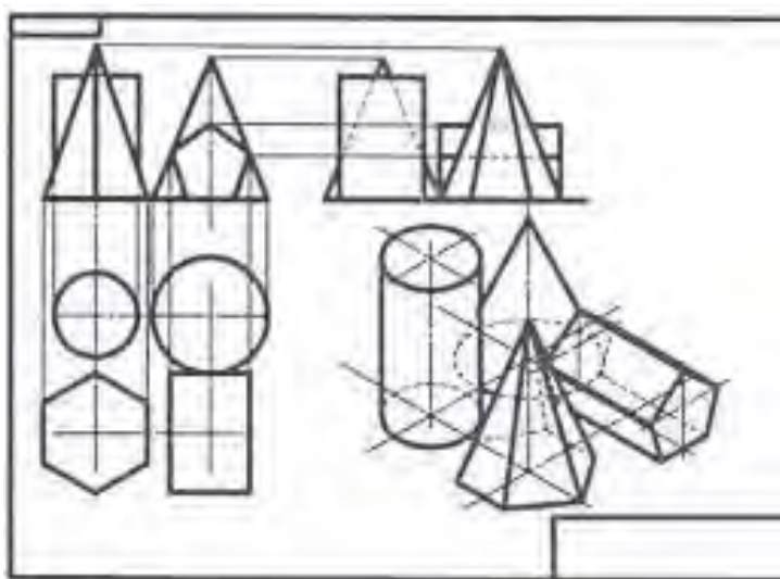
Рис. 2 Группа геометрических тел
