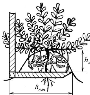
Впан – ковловчи панжа камраш кенглиги; h_n – ковлаш чукурлиги Рис. 2 Схема выкопки корневой части ореха лемехом с лемехом
