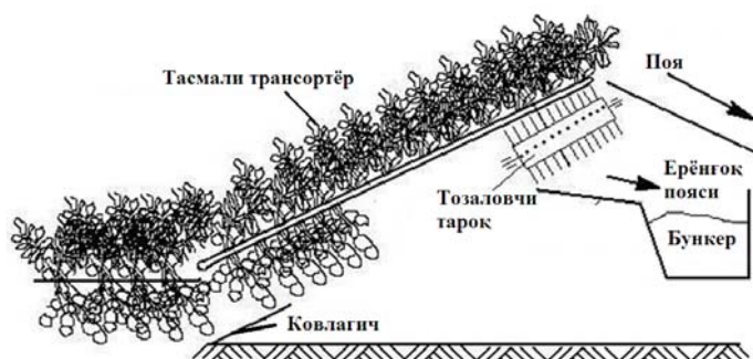
Рис. 3 Принципиальная схема процесса сбора орехов
