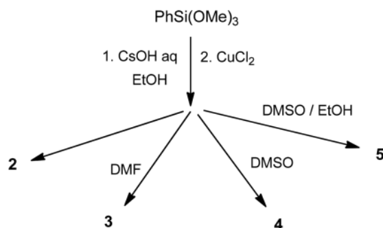
Рис. 2 Общая схема получения \text{Cu}_4\text{Cs}_4 -фенилсилсесквиоксанов 2-5
