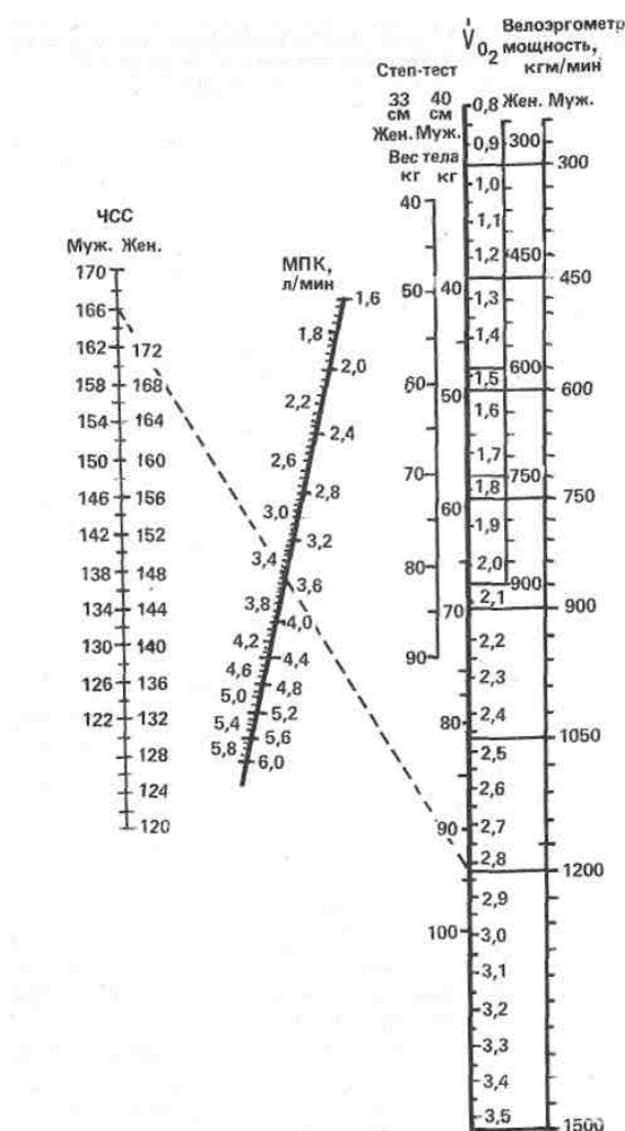
Рис. 1 Номограмма Астранда
