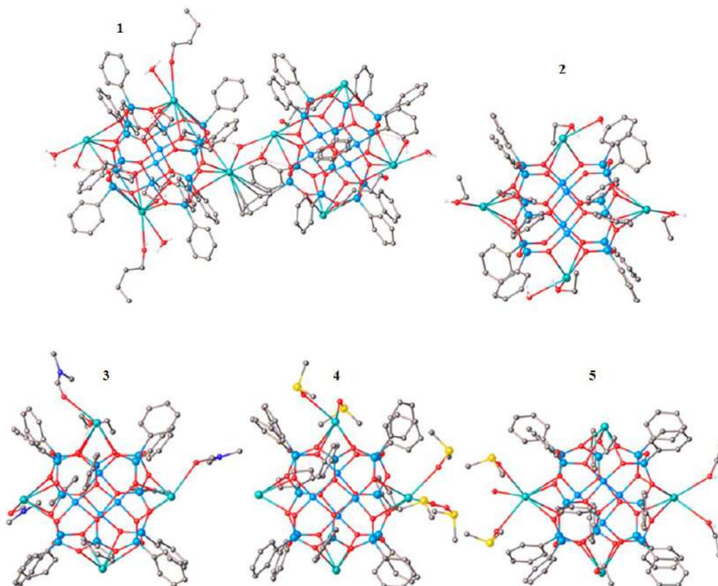
Рис. 3 Синтезированные \text{Cu}_4\text{Cs}_4 -фенилсилсесквиоксаны 1-5. Цветовой код: голубой, Cu; синий, Si; красный, O; бирюзовый, Cs; серый, C
