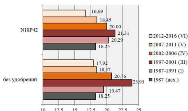
Рис. 1 Динамика содержания кислоторастворимых форм меди в пахотном слое почвы в зависимости от фона удобренности, мг/кг, HC P_{05}=1,27
