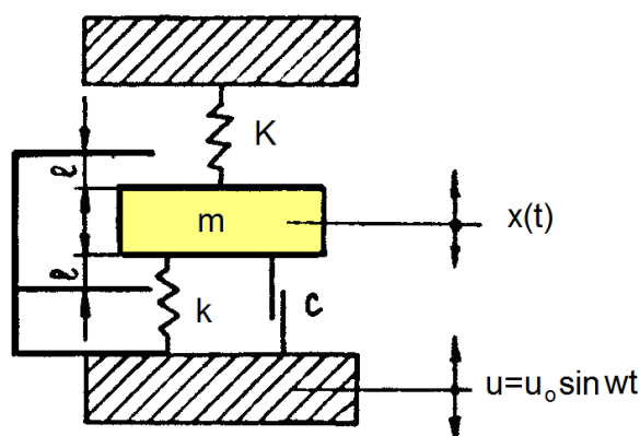
Рис.2 Расчетная схема дроссельного устройства с частотно-зависимым регулированием неупругого сопротивления
