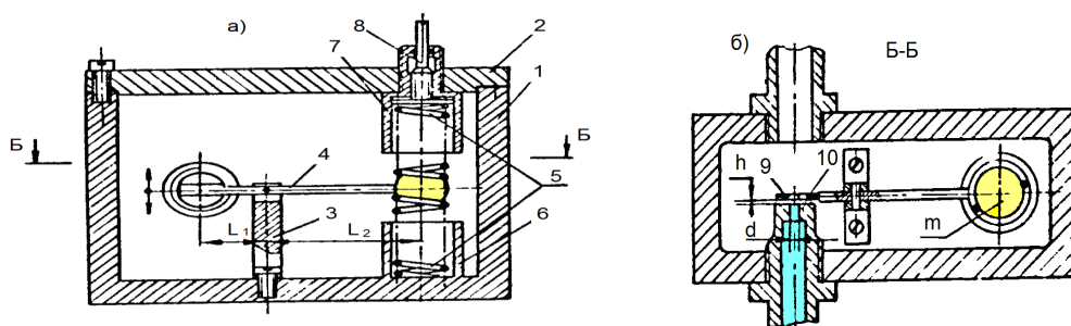
Рис. 3 Конструктивная реализация дроссельного устройства пневматической виброзащитной системы с частотно-зависимым регулированием неупругого сопротивления в виде язычкового резонатора
