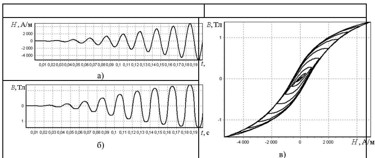
Рис. 4 Модель Джилса-Атертона (алгоритм JA ): а) – напряженность внешнего магнитного поля, б) – магнитная индукция в зависимости от времени, в) – петля гистерезиса по магнитной индукции
