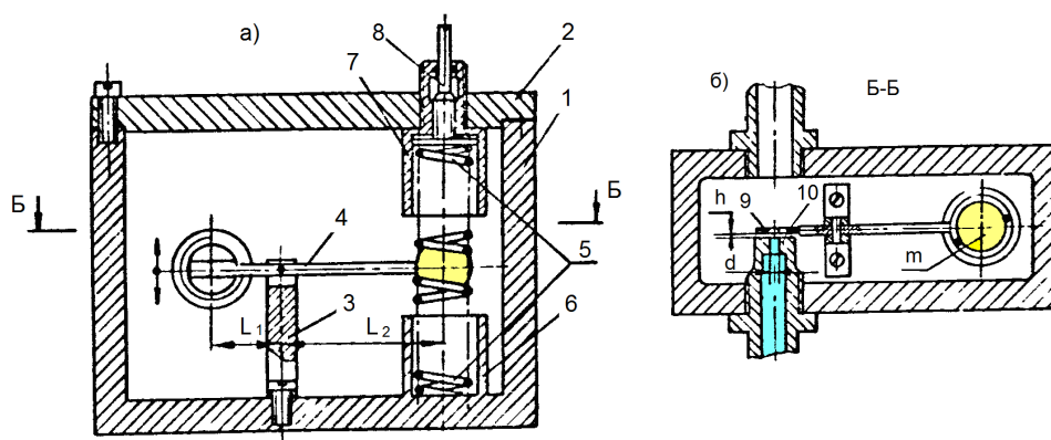
Рис. 2 Конструктивная реализация дроссельного устройства пневматической виброзащитной системы с частотно-зависимым регулированием неупругого сопротивления в виде язычкового резонатора
