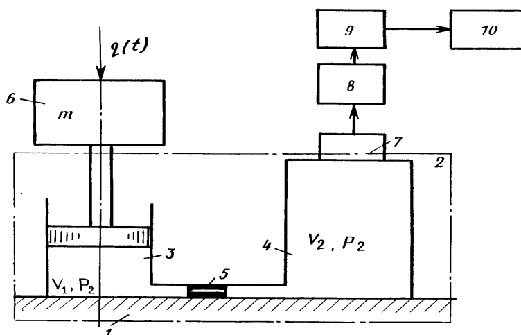
Рис.1 Схема стенда для определения пропускной способности нелинейного дроссельного устройства по методу опоражнения демпферной полости:
