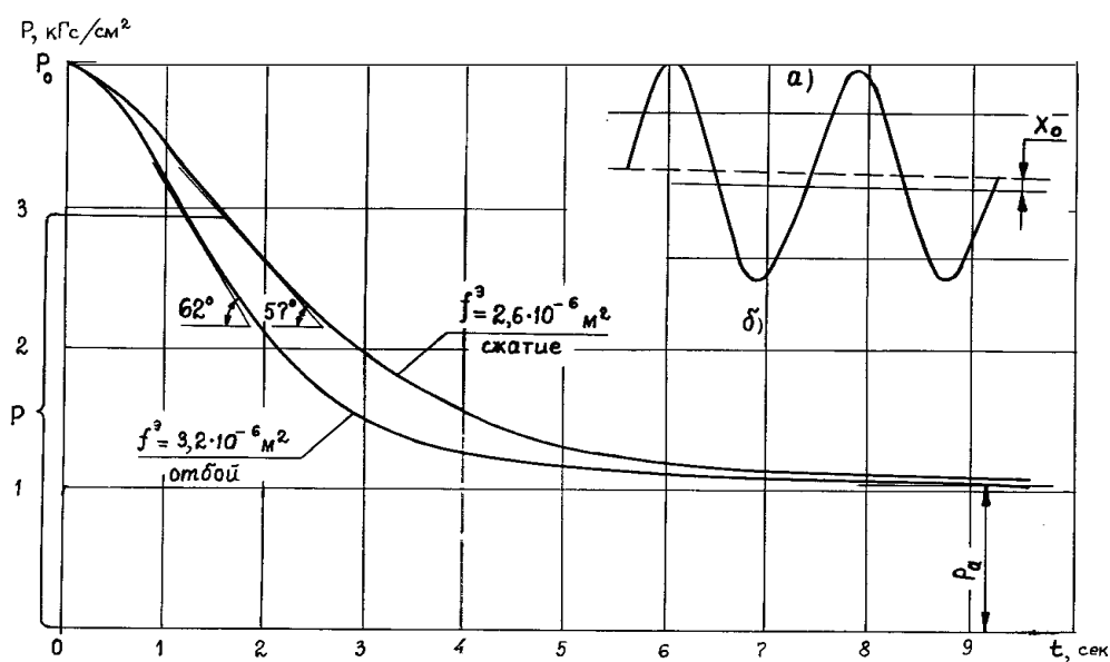
Рис.4 Экспериментальные характеристики нелинейного дроссельного устройства с частотно-зависимым сопротивлением дросселя в статическом состоянии, без вибрации
