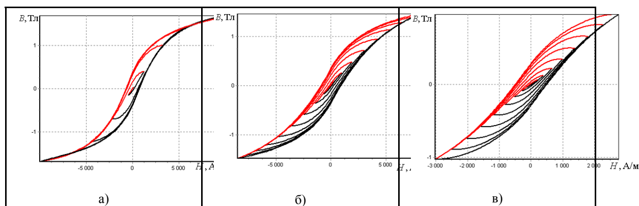
Рисунок 5. Петли гистерезиса в зависимости от частоты питающего тока:
