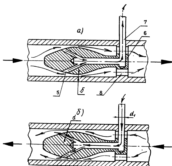
Рис. 2 Схемы движения газовых потоков пневмосистемы с полым обтекаемым дроссельным устройством: а) при ходе сжатия; б) при ходе отдачи
