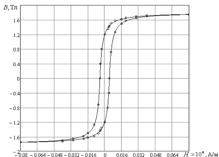
Рис. 2 Экспериментальная (точки) и рассчитанная петля (сплошная) стали Э330А
