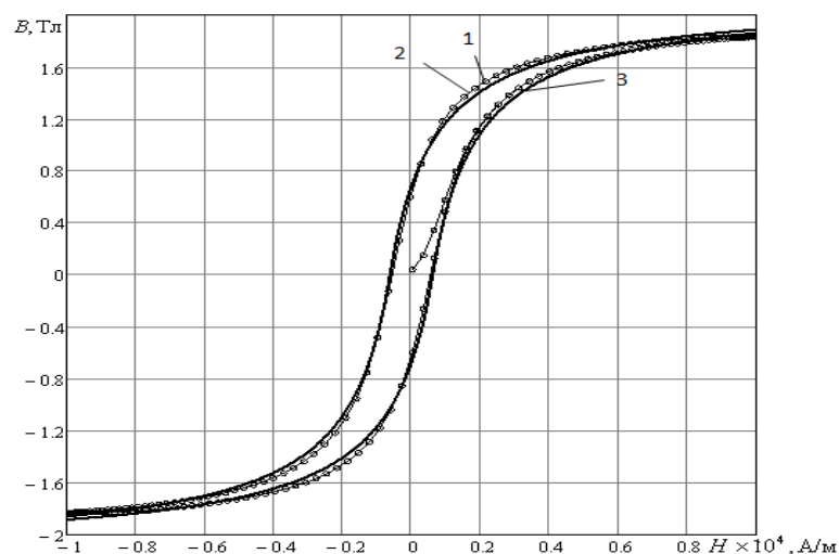
Рис. 3 Экспериментальная (точки) – 1, рассчитанная (сплошная) по алгоритму JA – 2, рассчитанная (жирная) по модели Чана – 3, петли гистерезиса плунжерной стали
