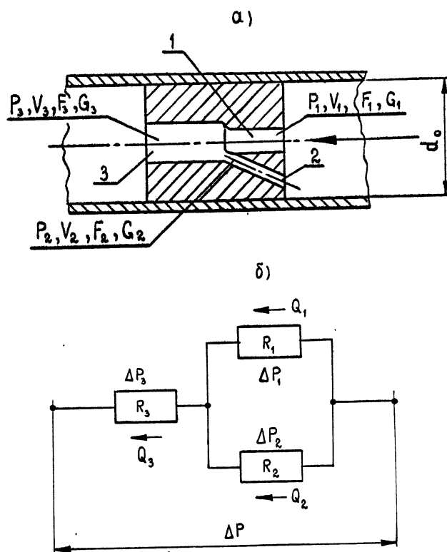
Рис. 3 Дроссельное устройство с несимметричной характеристикой неупругого сопротивления, работающее на принципе газовой эжекции: а) принципиальная схема эжектора; б) схема соединения пневмосопротивлений
