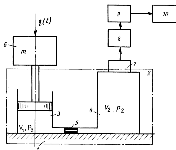
Рис. 4 Схема стенда для определения пропускной способности нелинейного дроссельного устройства по методу опоражнения демпферной полости: 1-основание, 2-пневмоподвеска, 3-рабочая камера, 4-демпферная камера, 5-нелинейное дроссельное устройство, 6-виброизолируемый объект, 7-датчик давления, 8-тензоусилитель, 9-осциллограф, 10-двухкоординатный самописец марки "Endim 620.01"
