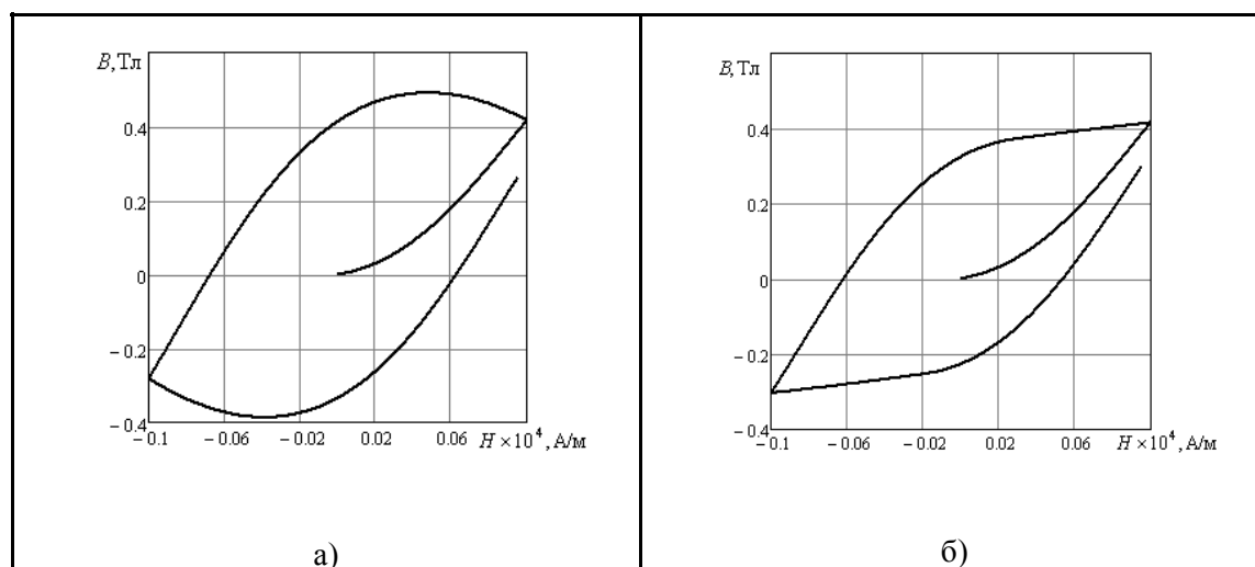
Рис.1 Модель Джилса-Атертона: а) при наличии отрицательной магнитной восприимчивости; б) при отсутствии отрицательной магнитной восприимчивости
