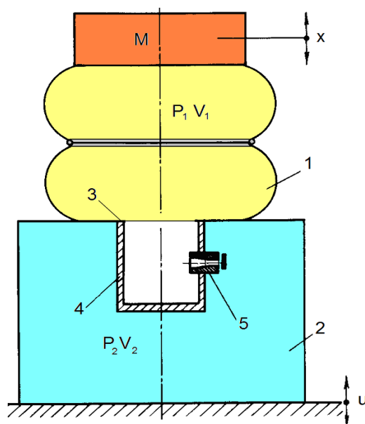
Рис.1 Общий вид пневматической виброзащитной системы
